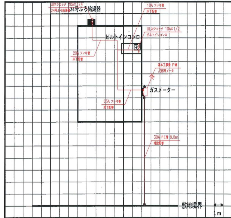
内管工事見積用平面図
