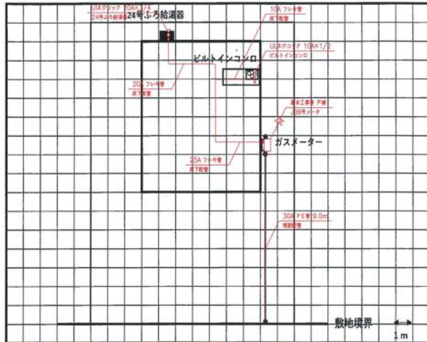
内管工事見積用平面図
